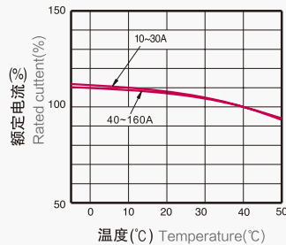
温度补偿曲线 Table.
