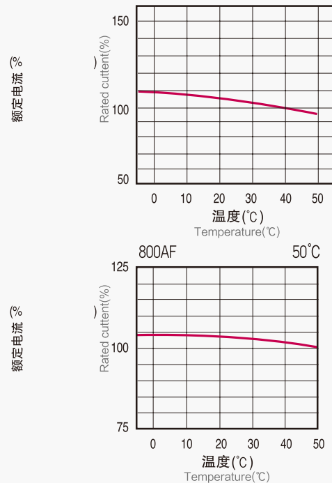
温度补偿曲线 Table.
