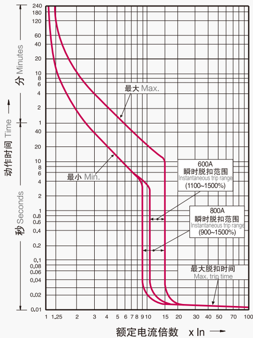
特性曲线 Spec.
