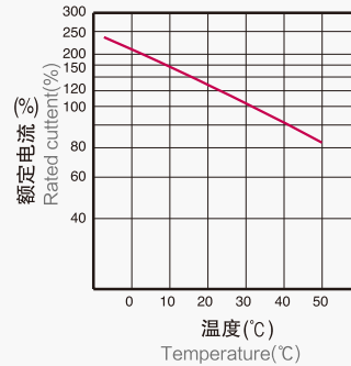
温度补偿曲线 Table.
