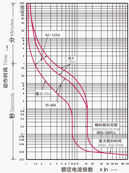
特性曲线 Spec.
